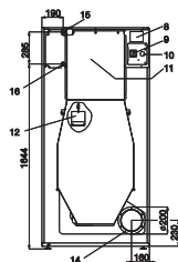
ЗАДНА СТРАНА Т 24 35 (МОДЕЛ ПАРА)
